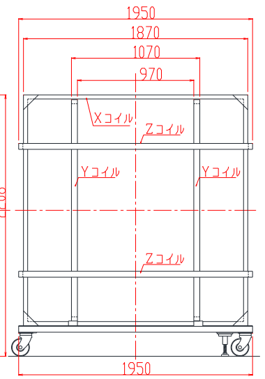
側面
